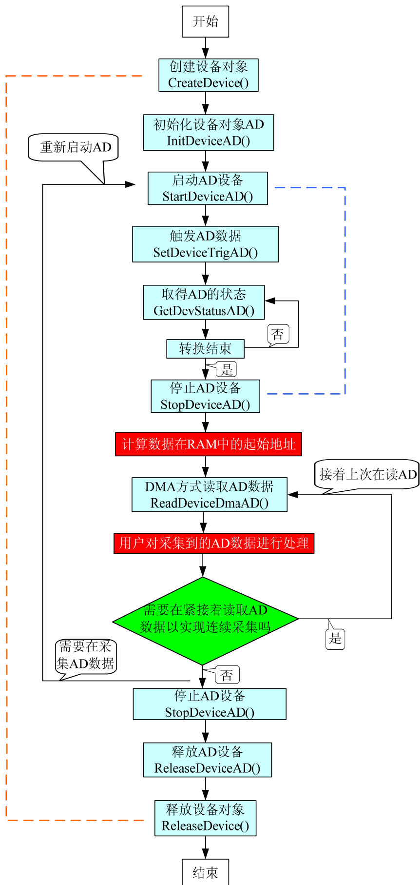
2.1.2 DMA 方式读取 AD 过程
